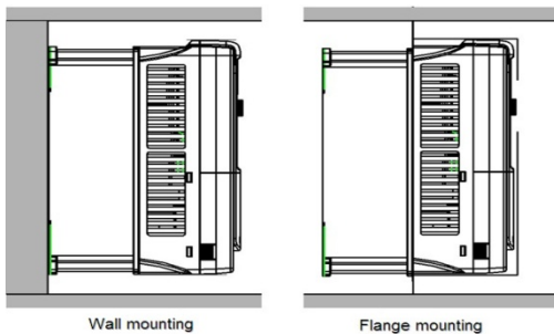
Рис. 3-1 Установка ПЧ
